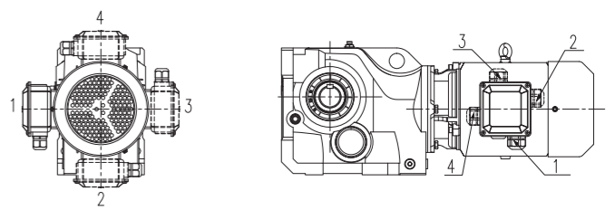
马达接线盒和进线孔位置 (视角:D1方位马达尾部)
