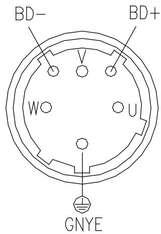
马达动力端插头 (100机座) Motor power end plug (100)
