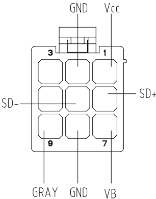
马达信号端插头 motor signal end
