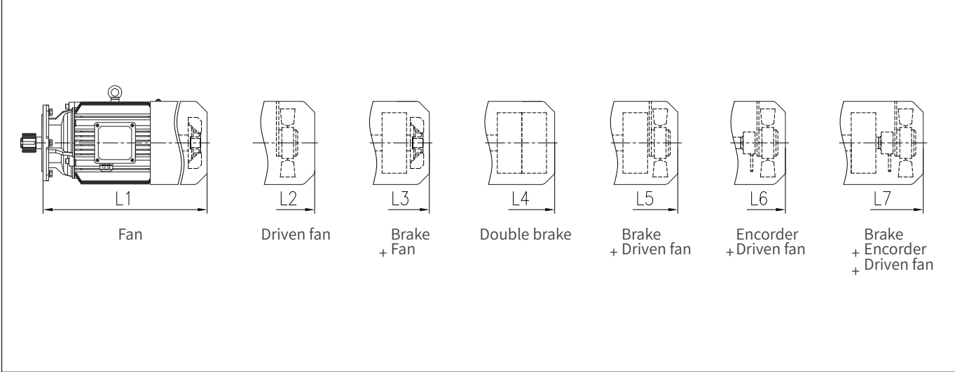
配S212对应马达 的外形尺寸图表 Corresponding motor dimension table for S212
